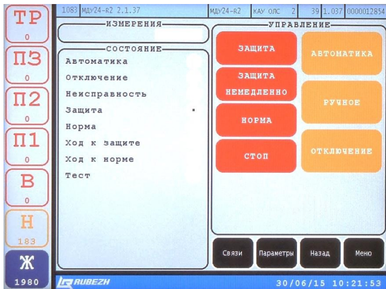
Рисунок 52 – Окно Компонент МДУ24-Р2
