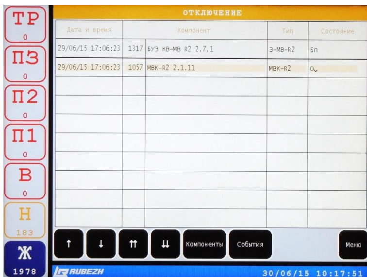
Рисунок 47 – Окно ОТКЛЮЧЕНИЕ
