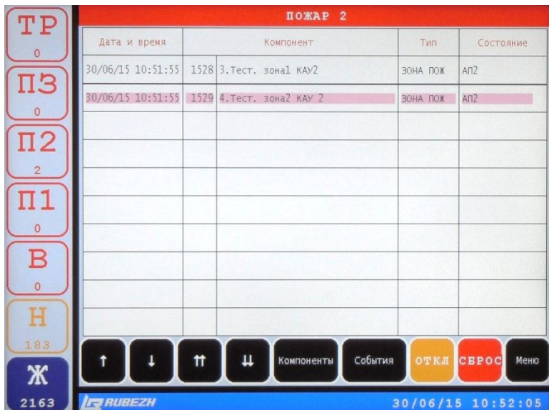
Рисунок 41 – Окна ПОЖАР 1 , ПОЖАР 2
