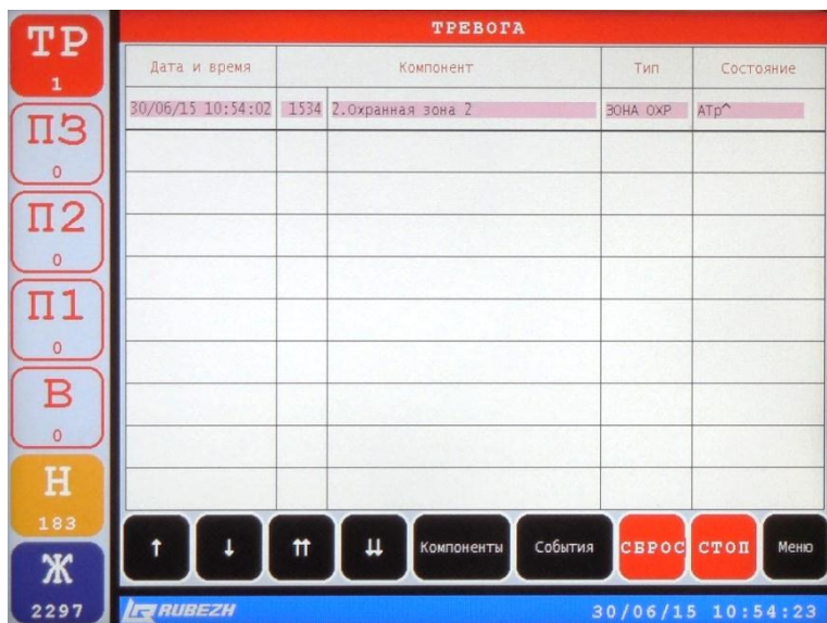
Рисунок 44 – окно ТРЕВОГА
